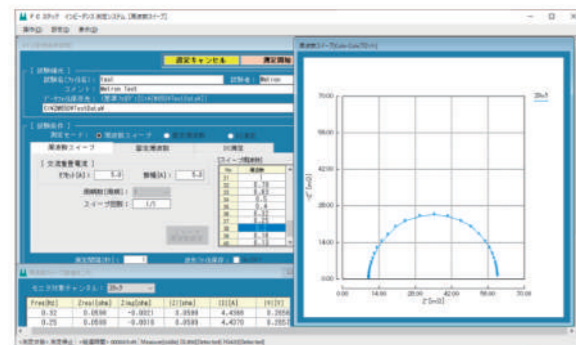
周波数スイープモード Frequency sweep mode
