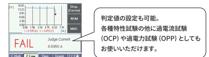
Sweep CRモード判定例(例:過電流特性試験)
