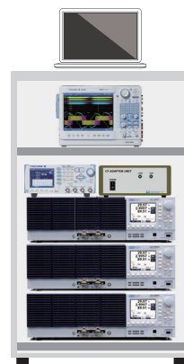
燃料電池インピーダンス測定システム
